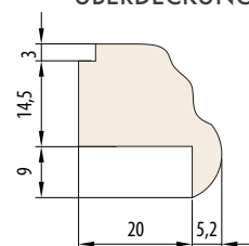
ÜBERDECKUNGS-GLASLEISTE
