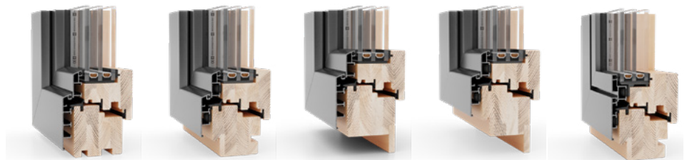
Gemini Classic Standardprofil (ohne Fensterbankfräsung)
