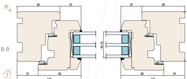
SYSTEM NATURO 92 Äußere Fensterbankfräsung
