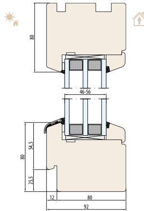
SYSTEM NATURO 92-Fix Äußere Fensterbankkräsung
