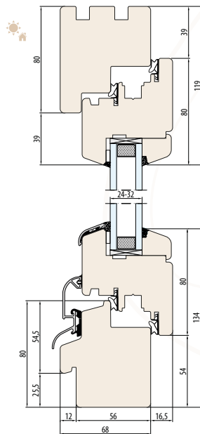
SYSTEM NATURO 68 Äußere Fensterbankfräsung
