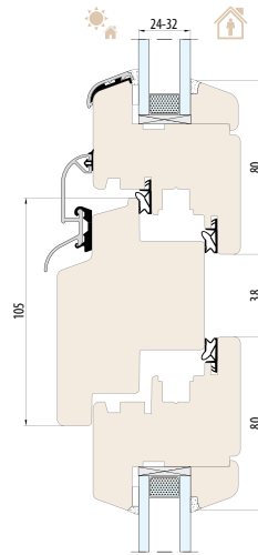
SYSTEM NATURO 68 Querschnitt 105 mm
