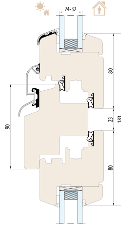
SYSTEM NATURO 68 Querschnitt 90 mm
