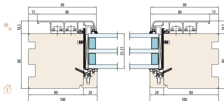
HORIZONTALSCHNITT B-B
