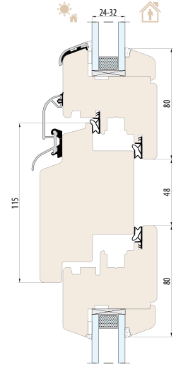
SYSTEM NATURO 68 Querschnitt 115 mm
