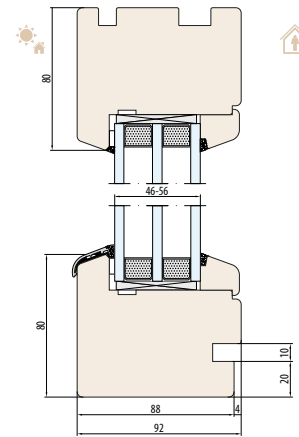
SYSTEM NATURO 92-Fix Innere Fensterbankkräsung
