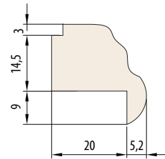
ÜBERDECKUNGS-GLASLEISTE
