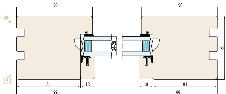
SYSTEM ESPERIA LIFE 80-Fix HORIZONTALSCHNITT B-B
