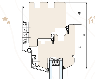
VERTIKALSCHNITT A-A
