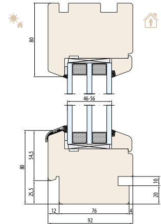
SYSTEM NATURO 92-Fix Innen- und Außenfensterbankkräsung
